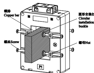
压盘固定 Pressing tray fix
