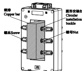
压盘固定 Pressing tray fix
