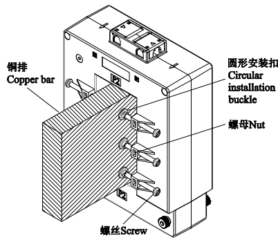
压盘固定 Pressing tray fix
