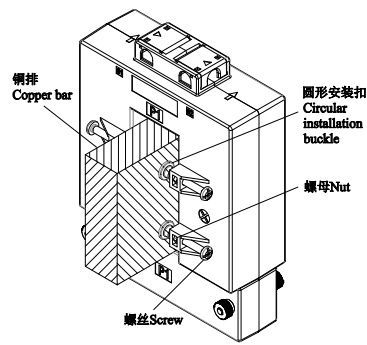
压盘固定 Pressing tray fix
