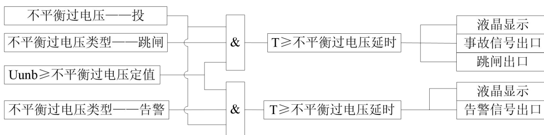
图 3-10: 不平衡过电压保护动作逻辑图
