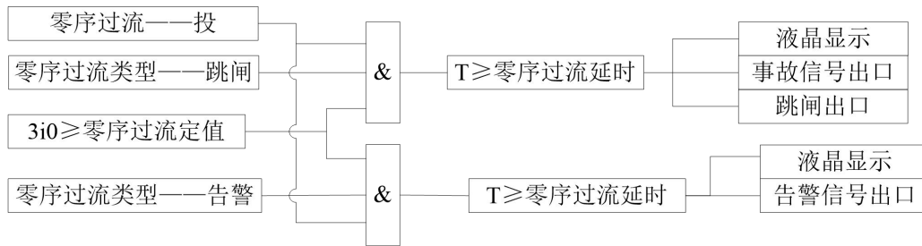
图 3-6：零序过流保护动作逻辑图
