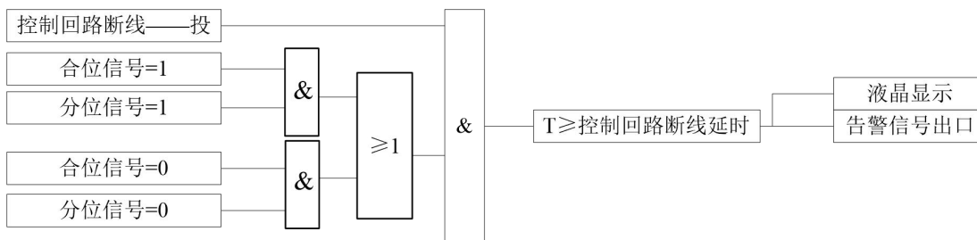
图 3-12: 控制回路断线保护动作逻辑图
