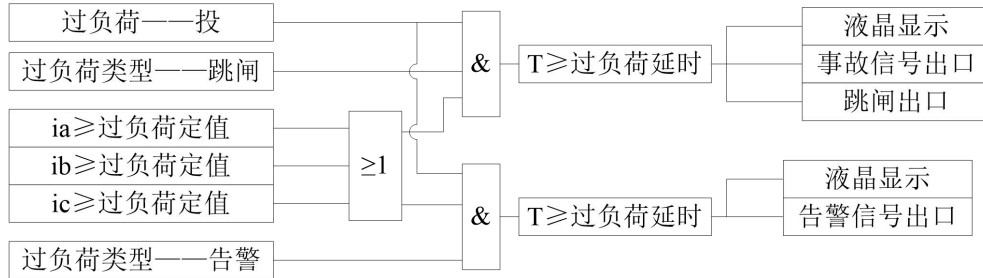
图 3-5：过负荷保护动作逻辑图
