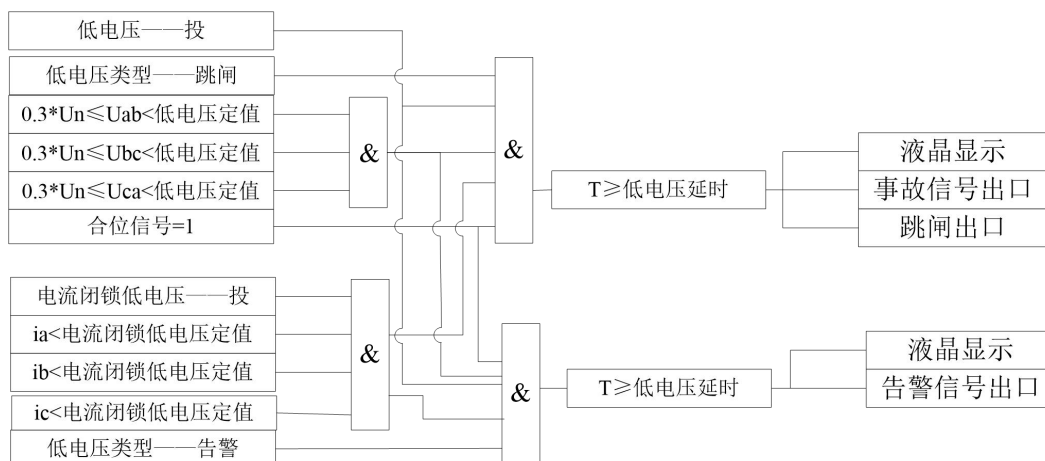
3-9: 低电压保护逻辑框图
