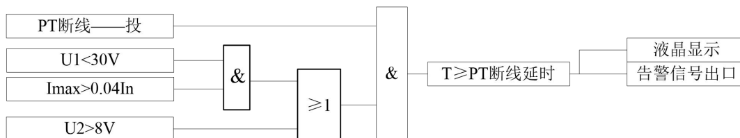
图 3-11: PT 断线保护动作逻辑图
