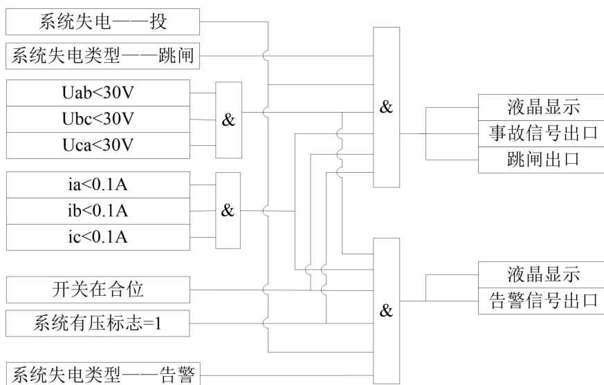
图 3-13：系统失电保护动作逻辑图
