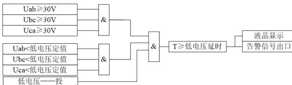
图 3-2：低电压保护逻辑框图
