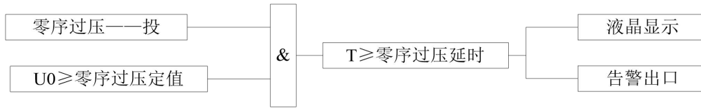
图 3-4：母线零序过压保护逻辑框图
