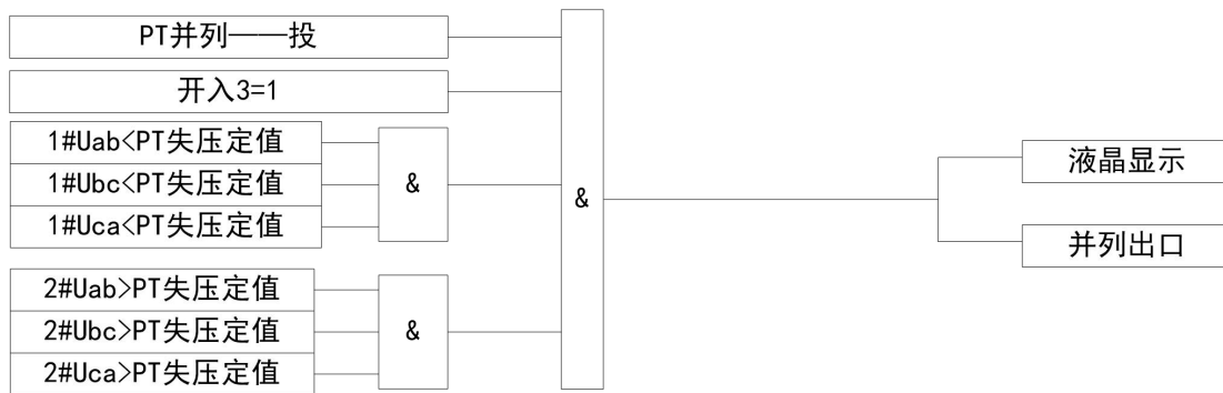
图 3-5：II 母 PT 并列保护逻辑框图
