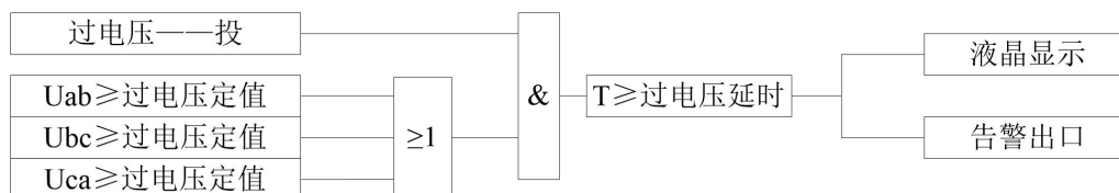
图 3-1：过电压保护逻辑框图
