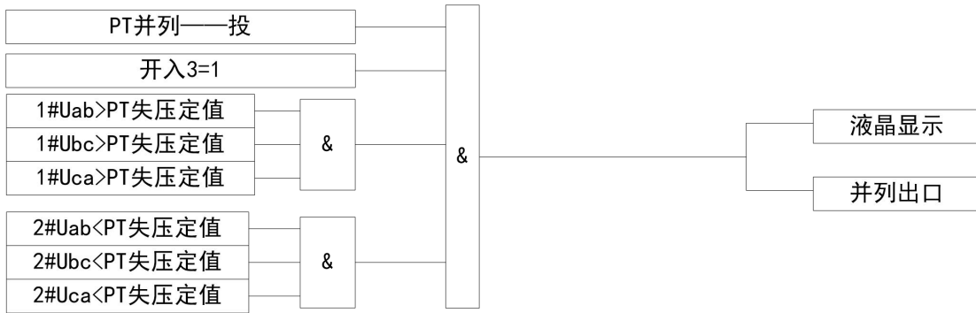
图 3-6: I 母 PT 并列保护逻辑框图
