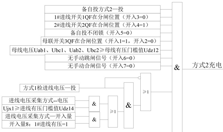
图 3-11: 备自投方式 2 充电逻辑图
