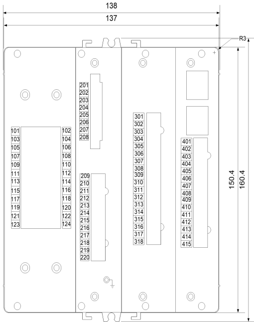
背板示意图
