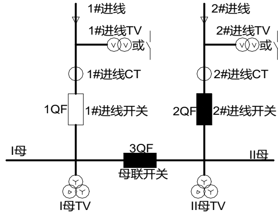
图 3-10: 备自投方式 2 运用的场合
