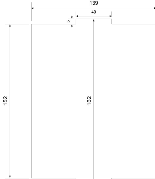
开孔尺寸图
