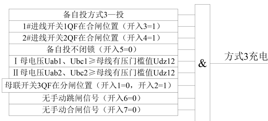
图 3-14：备自投方式 3 的充电逻辑图
