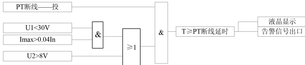
图 3-14: PT 断线保护动作逻辑图
