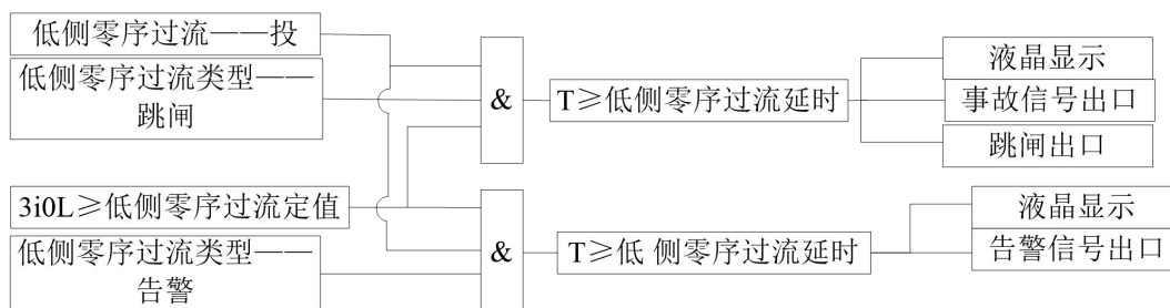
图 3-9：零序过流保护动作逻辑图
