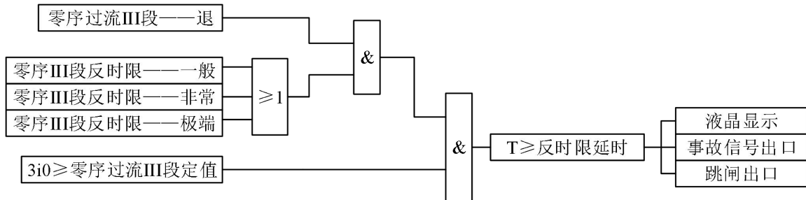
图 3-7：零序 III 段反时限保护动作逻辑图
