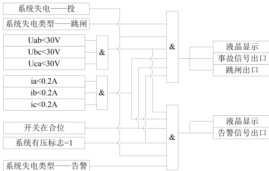
图 3-16：系统失电保护动作逻辑图
