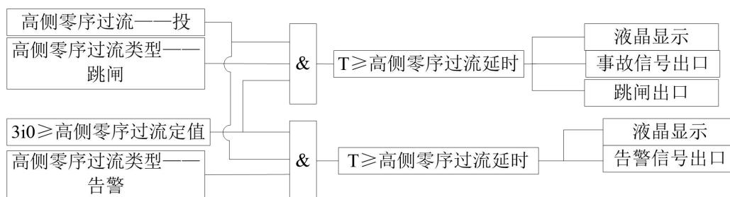
图 3-8：零序过流保护动作逻辑图
