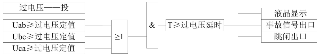
图 3-11: 过电压保护动作逻辑图
