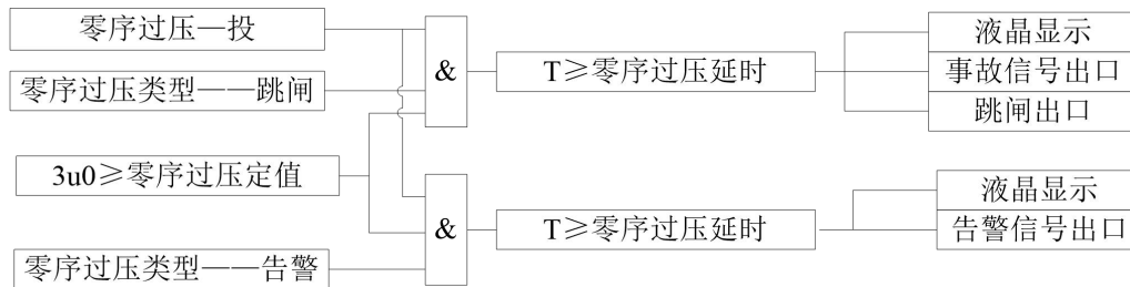
图 3-13: 零序过压保护动作逻辑图
