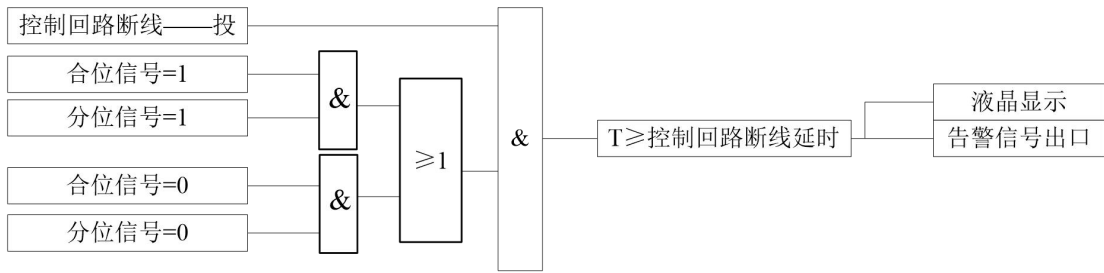
图 3-15：控制回路断线保护动作逻辑图
