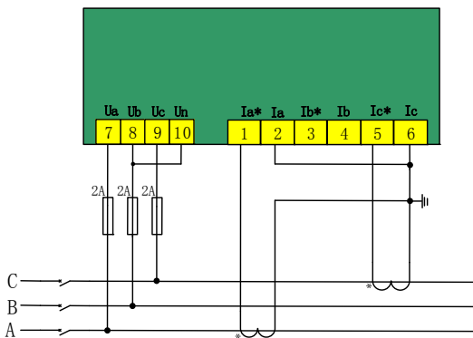
三相三线，无 PT,2CT
