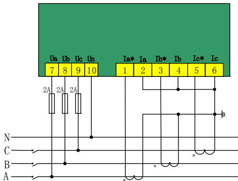
三相四线系统，无 PT,3CT
