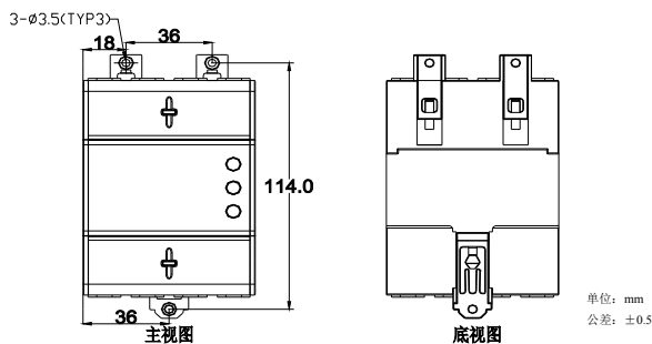
M3螺丝固定安装方式
