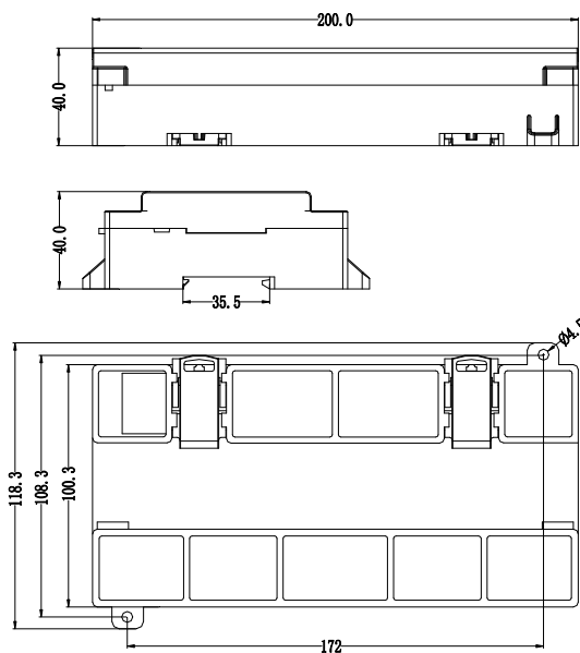
尺寸图 (单位: mm, 公差: \pm 0.5 )
