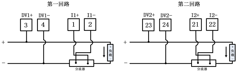
分流器接负端
