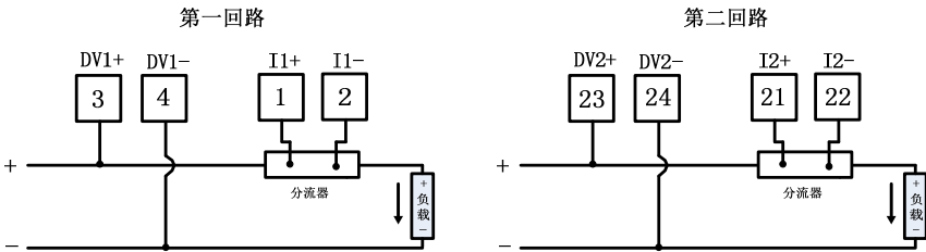
分流器接正端
