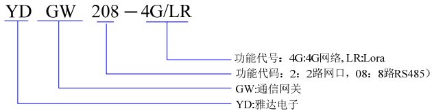
图 1.2 通信网关型号定义图
